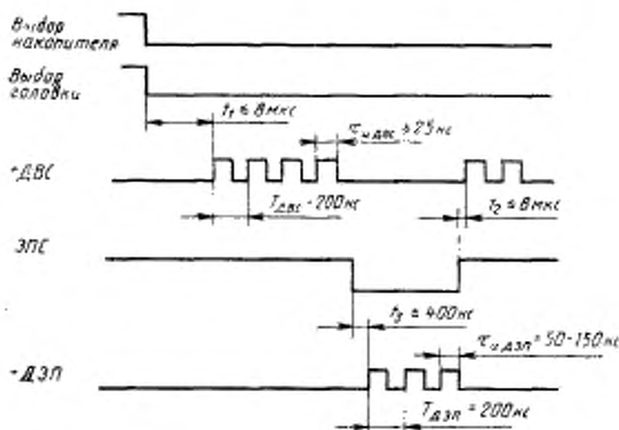
Временные соотношения сигналов ЗПС, ДЗП, ДВС
