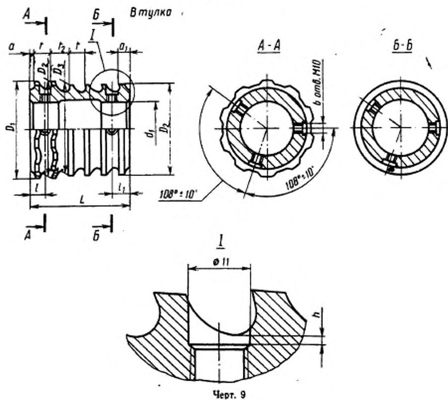
Втулка
