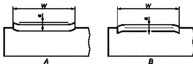
Рисунок 3 — Профиль поверхности
