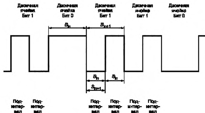
Рисунок 11 — Изменение промежутка между переходами потока
