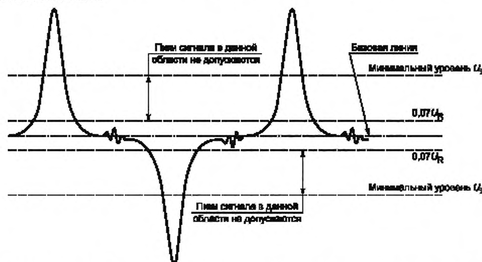
Рисунок 10 — Присутствие нежелательных пиков в форме сигнала
