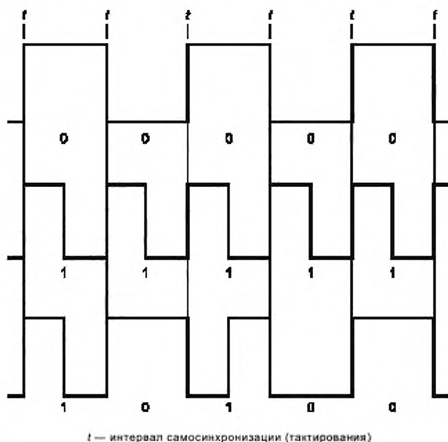
Рисунок 8 — Пример двухчастотного синфазного кодирования
