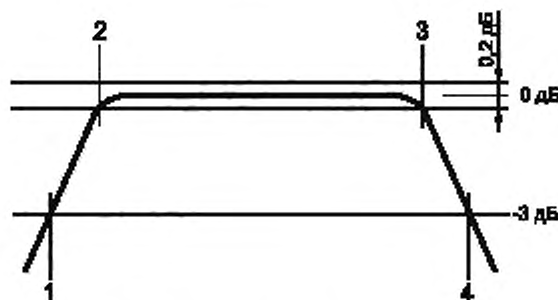
Рисунок В.1 — Характеристики полосового фильтра
