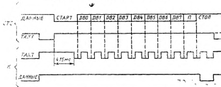
Передача данных от сопрягаемого технического средства клавиатуре при 11-битном обмене
