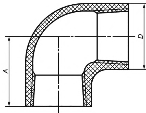
Рисунок 4 — Отвод с углом поворота 90°
