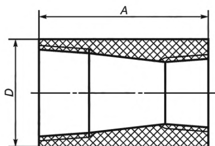
A — длина муфты; D — наружный диаметр
