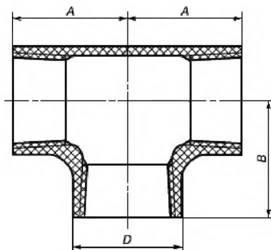
Рисунок 8 — Равнопроходной тройник
