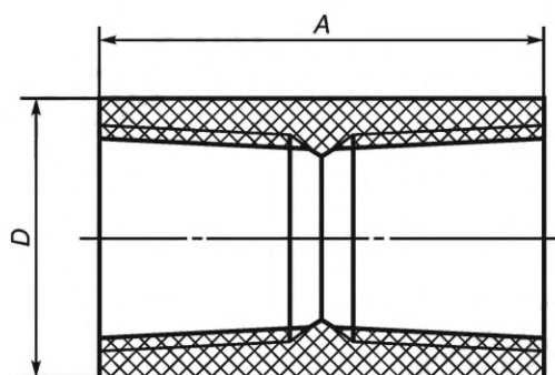
A — длина муфты; D — наружный диаметр
