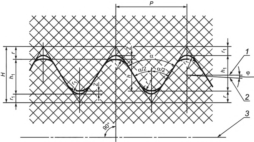
1 — линия, параллельная оси резьбы; 2 — линия среднего диаметра резьбы; 3 — ось резьбы; P — шаг резьбы (измеряют параллельно оси резьбы); H — высота исходного профиля; h_1 — высота профиля; h — рабочая высота профиля; \alpha — угол профиля; Z — зазор; \phi — угол наклона; r , r_1 — радиус закругления
