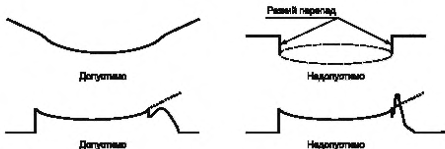
Рисунок 4 — Примеры профилей поверхности
