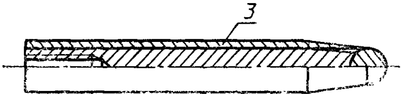
1 — латунный стержень с наплавным стальным шариком; 2 — изолирующее покрытие; 3 — разрядный электрод в сборке.
