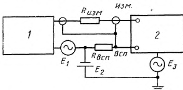
Блок-схема определения наибольших допускаемых изменений погрешностей преобразователей по выходному сигналу
