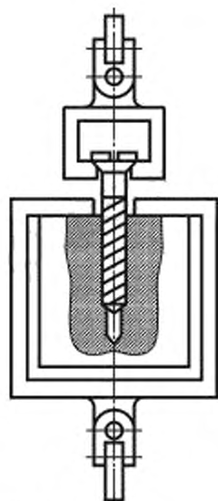
Рисунок 1 — Схема выдергивания шурупа из пласти плиты Рисунок 2 — Схема выдергивания шурупа из кромки плиты
