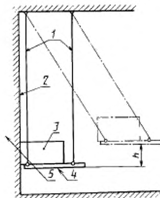
Схема маятникового прибора
