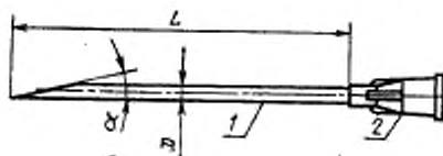
1—трубка иглы; 2—головка иглы
