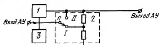
1 — АУ; 2 — аттенуатор; 3 — электронный милливольтметр; П — переключатель
