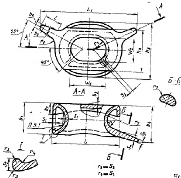
Размеры, мм
