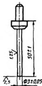
Рисунок 1 — Пестик к прибору Вика
