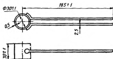
Рисунок 2 — Кольцо Ле-Шателье
