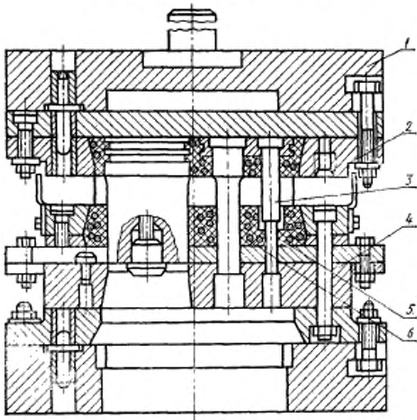
1—блок; 2—пакет последовательного действия; 3—пистон; 4—матрица; 5—самотвердеющая акриловая пластмасса; 6—арматурный каркас
