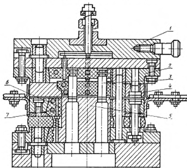
1—блок; 2—пакет совмещенного действия; 3—пуансон; 4—матрица; 5—пуансон-матрица; 6—самотвердеющая акриловая пластмасса; 7—проводящий каркас
