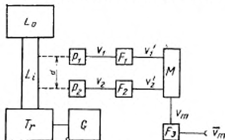
Схема измерений методом потока мощности
