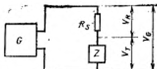
Основная схема метода трех вольтметров
