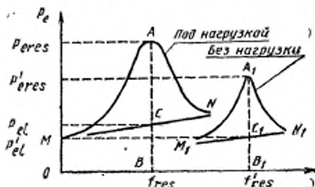
Частотные характеристики электрической входной мощности преобразователя
