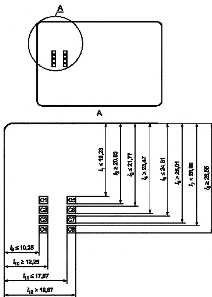
Рисунок 2 — Расположение контактов
