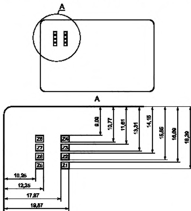
Рисунок В.1 — Расположение возможных проводящих зон
