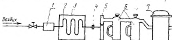
1—осушитель воздуха; 2—контролируемый элемент; 3—сушильный шкаф; 4—зажим; 5—реометр; 6—трубки Нессбита; 7—компрессор
