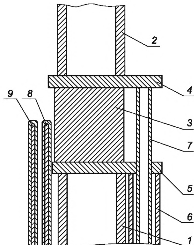
1 — нижний штамп; 2 — верхний штамп; 3 — образец; 4 — верхняя прокладка; 5 — нижняя прокладка; 6 и 7 — трубы, передающие деформацию; 8 — термопара для измерения температуры образца; 9 — термопара для управления печью
