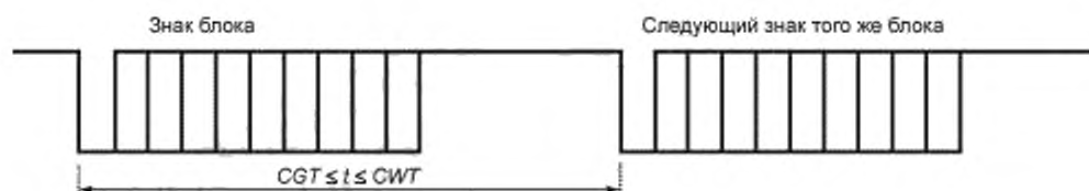
Рисунок 21 — Время ожидания знака в пределах блока
