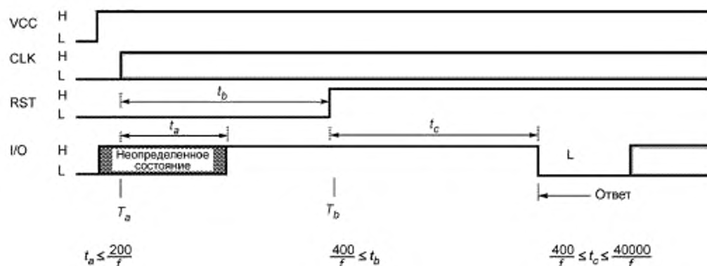
Рисунок 1 — Активация и «холодное» восстановление
