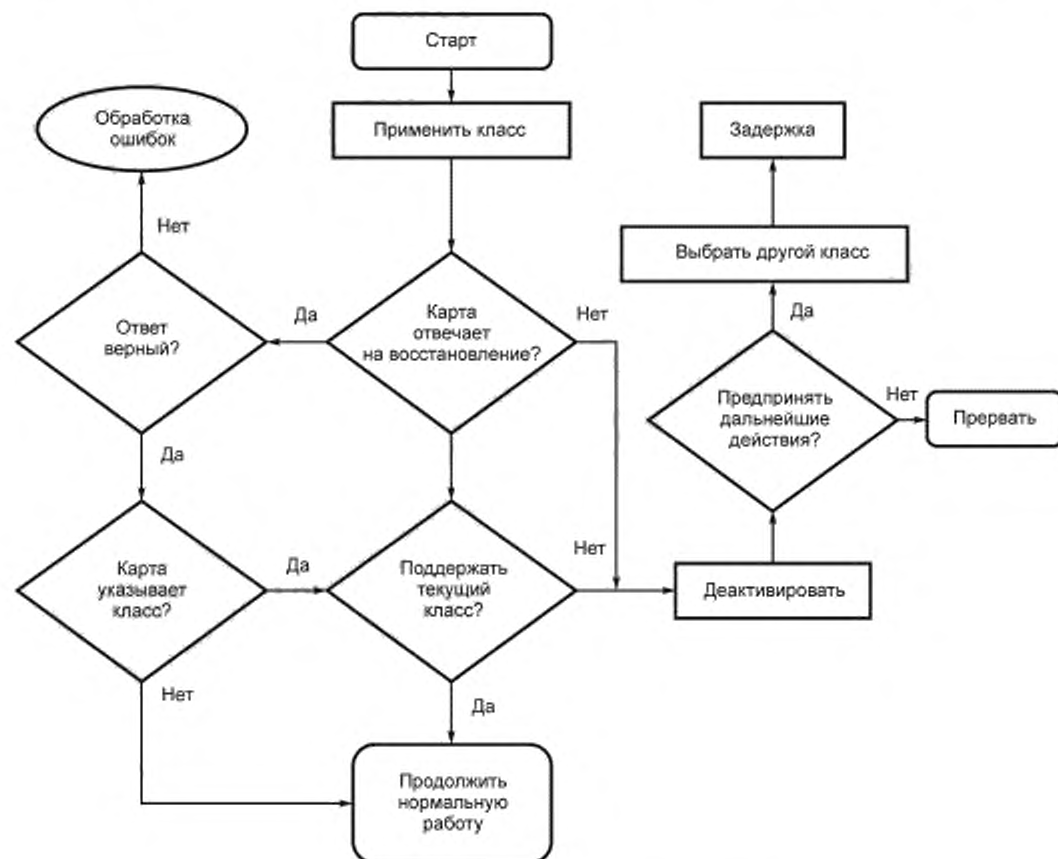
Рисунок 3 — Выбор класса устройством сопряжения
