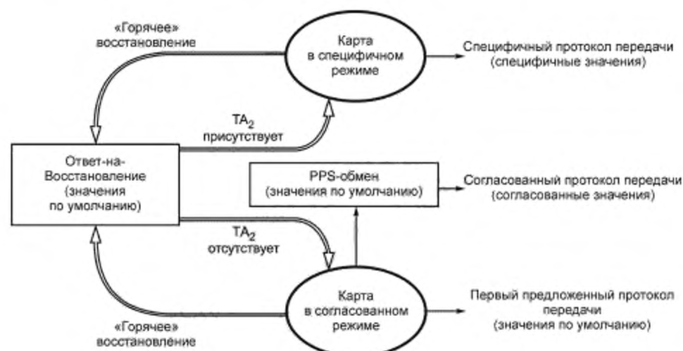
Рисунок 4 — Выбор параметров передачи и протокола
