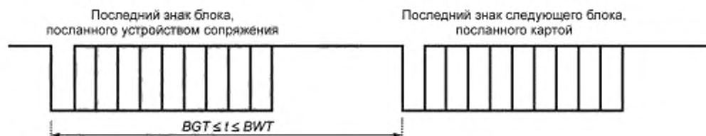
Рисунок 22 — Время ожидания блока
