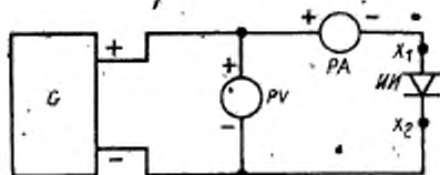
G — источник постоянного (немодулированного или модулированного) напряжения; PV — измеритель напряжения; PA — измеритель тока; II — испытуемый индикатор; X_1 и X_2 — контакты подключения испытуемого индикатора
