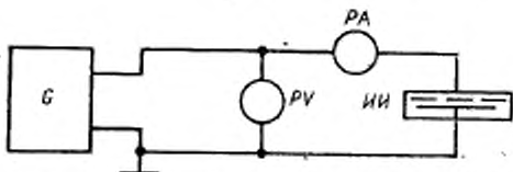
G — регулируемый источник переменного напряжения; PV — вольтметр переменного напряжения; PA — микро- амперметр переменного тока; ИИ — испытуемый инди- катор
