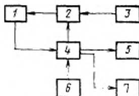
1 — фотоприемное устройство; 2 — испытуемый индикатор; 3 — источник света; 4 — устройство управления; 5 — осциллограф; 6 — источник управляющего напряжения индикатора; 7 — измеритель временных интервалов
