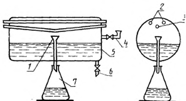
1 — воронка; 2 — нагреватель; 3 — холодильник; 4 — бран для заливки кислоты; 5 — колба; 6 — кран для слива кислоты; 7 — колба
