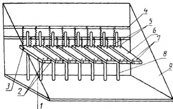
1 — электрод; 2 — токовод; 3 — винт-фиксатор держателя; 4 — штифт-пружина; 5 — гибкий провод; 6 — держатель; 7 — отверстие для электрода; 8 — стойка; 9 — корпус из оргстекла
