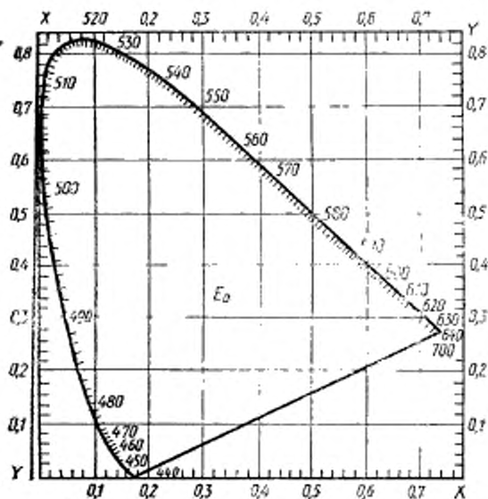
ЦВЕТОВОЙ ГРАФИК СИСТЕМЫ МКО
