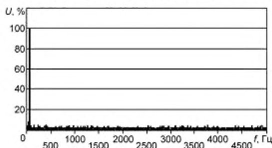
Спектр частот напряжения на выходе преобразователя — инвертора напряжения типа В f_1 равен 50 Гц, f_{ср} — 4,5 кГц
