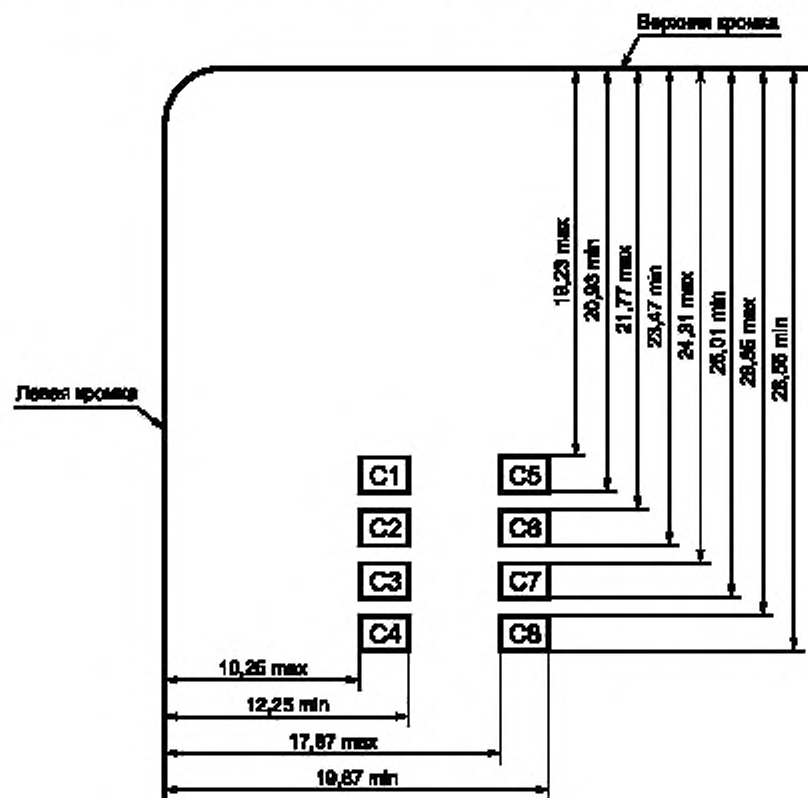
Рисунок 2 — Расположение контактов
