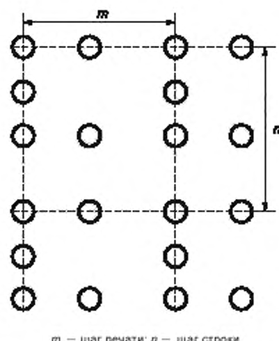
Рисунок 2 — Геометрические расположения символов шрифта Брайля на носителе данных
