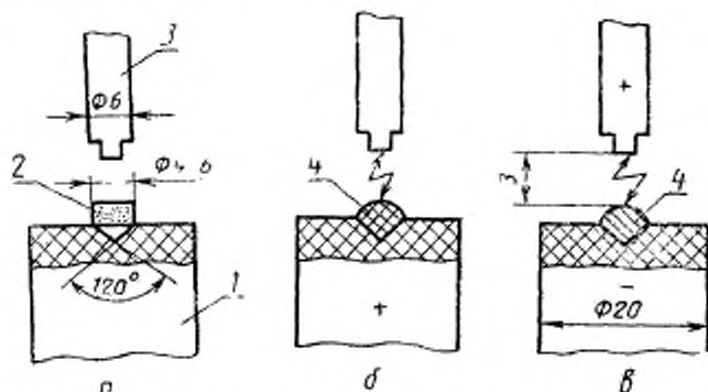
1 — графитовый электрод-подставка; 2 — таблетка пробы или стандартного образца; 3 — графитовый электрод; 4 — капля расплава. а — до экспонирования; б — при анодной полярности таблетки; в — при катодной полярности таблетки
