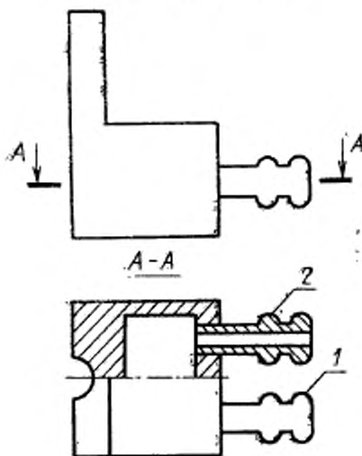
1 — штуцер для входа охлаждающей воды, 2 — штуцер для выхода охлаждающей воды.
