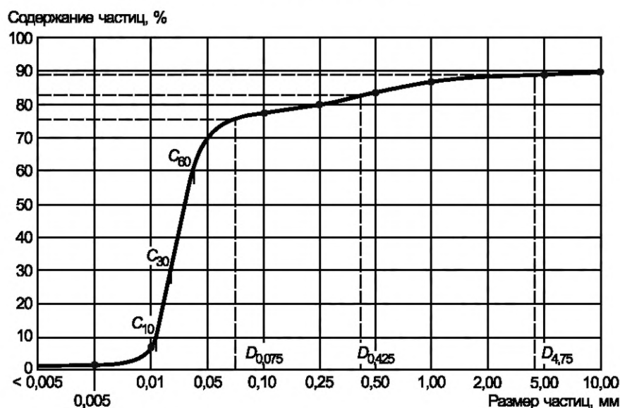
Рисунок Е.2 — Кумулятивная кривая гранулометрического состава
