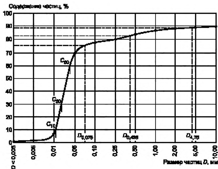
Рисунок Е.2 — Кумулятивная кривая гранулометрического состава
