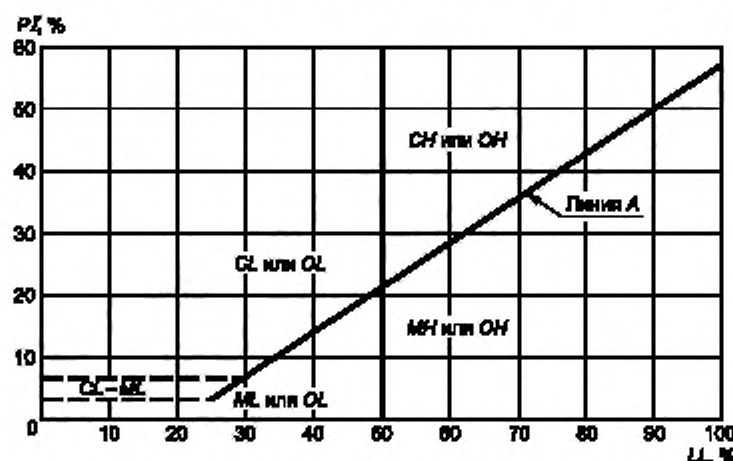
Рисунок Е.3 — График пластичности грунтов (plasticity chart)
