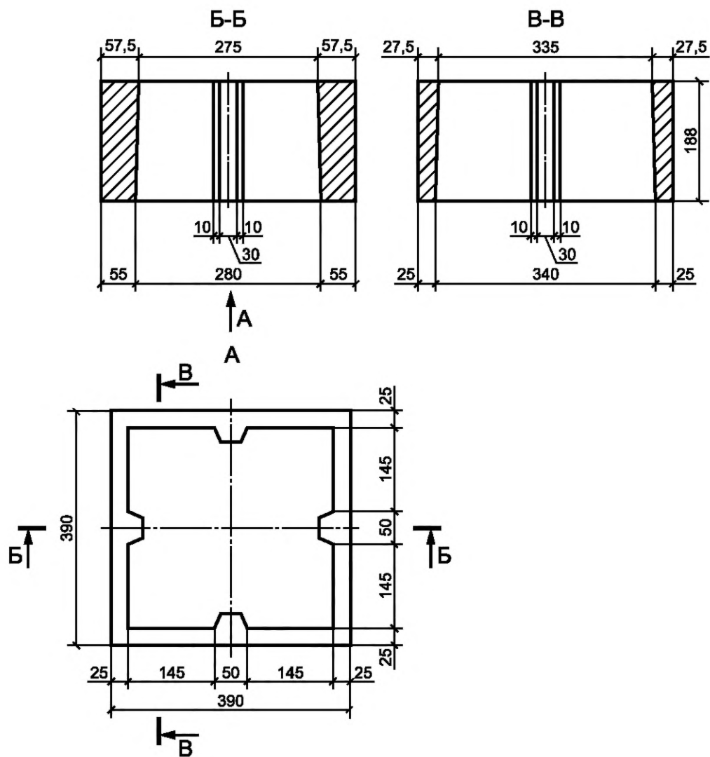
Рисунок А.19 — Камень для дымовой трубы
