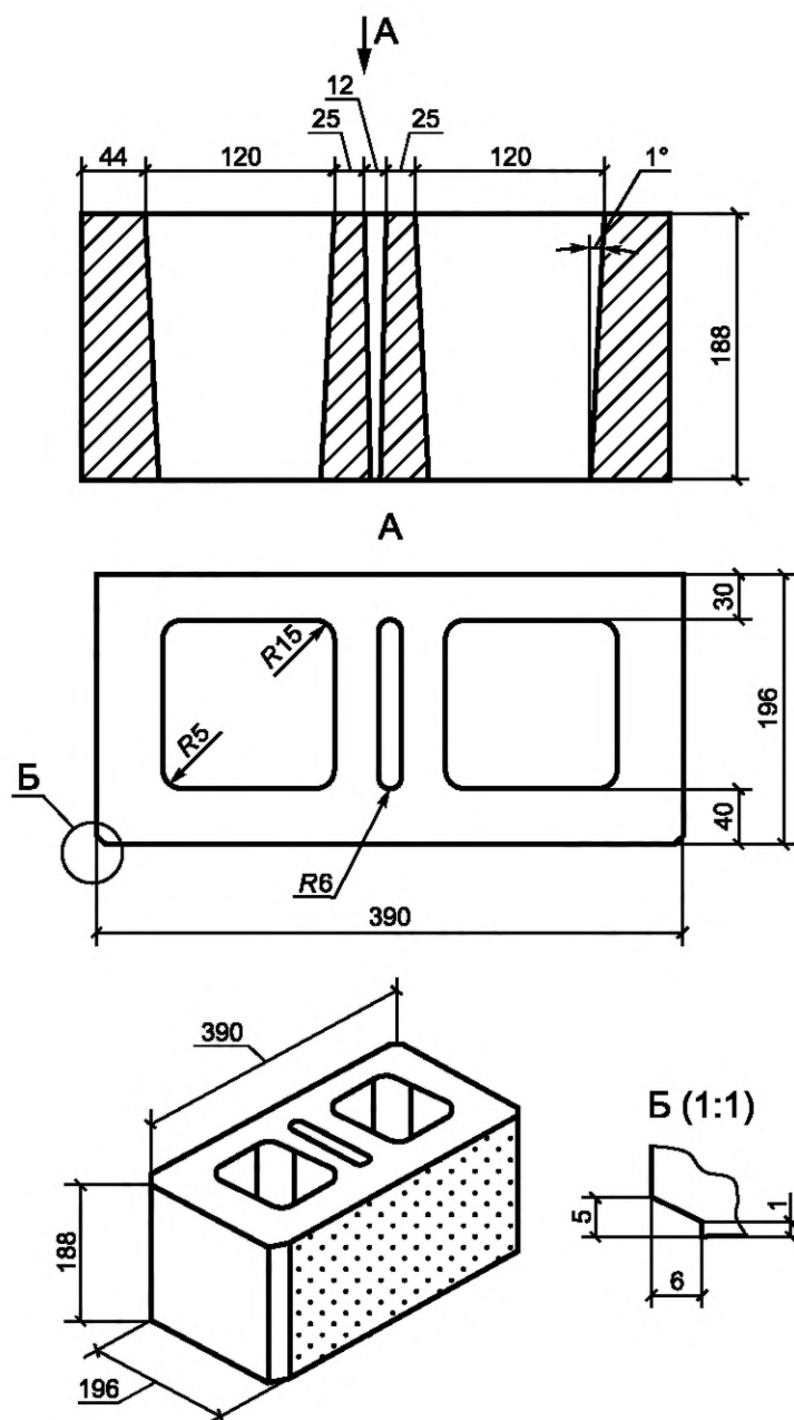
Рисунок А.12 — Камень лицевой декоративный угловой
