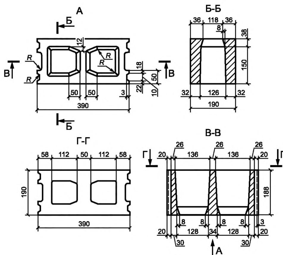
Рисунок А.15 — Камень стеновой рядовой
