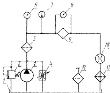
Схема стенда для определения гидравлической характеристики
