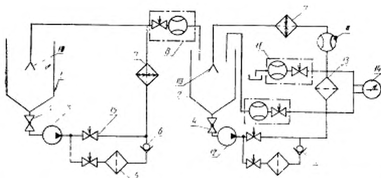
Схема испытательного стенда для определения характеристик фильтрации
