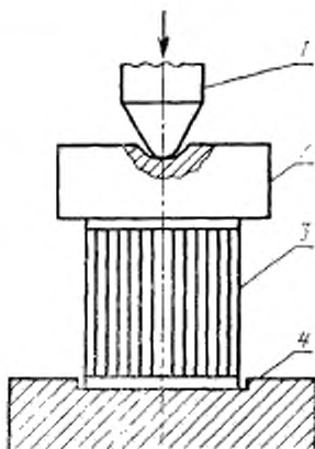
1—сжимающий штифт; 2—сжимающая шайба; 3— фильтроэлемент; 4—основание
