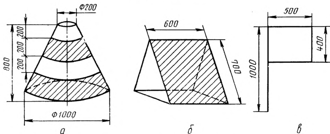
а—усеченный конус; б—призма; в—флажок
