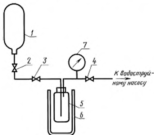
Схема подготовки сжиженного моноэтиламина
