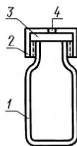
1 — сосуд; 2 — крышка; 3 — резиновая мембрана; 4 — отверстие в крышке
