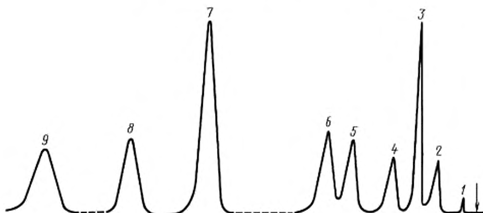
Хроматограмма искусственной смеси этиламинов
