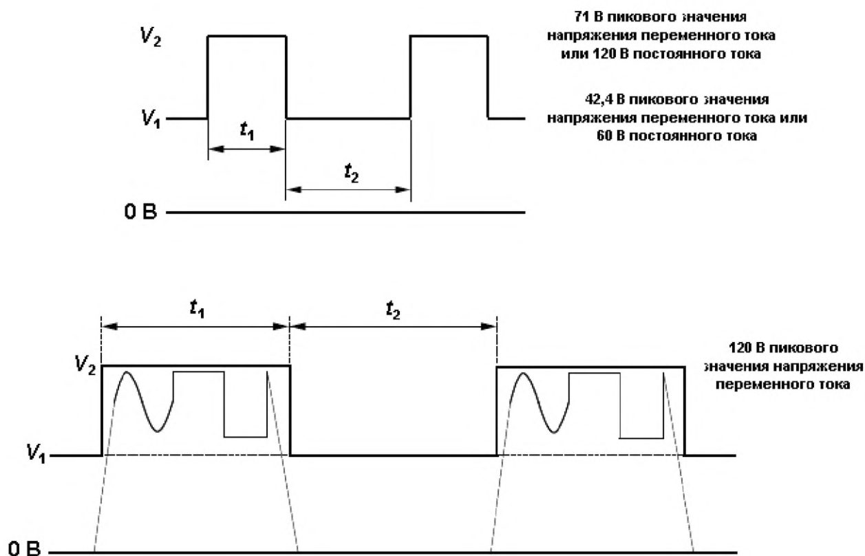
Рисунок 2Е.1 — Напряжения в БСНН цепях в условиях единичной неисправности при одиночном импульсе выше V_1
