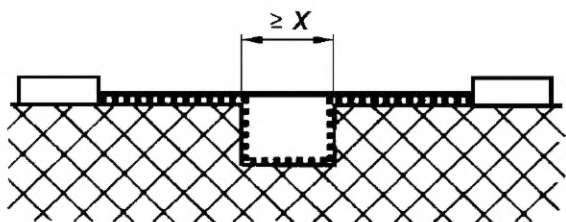
Рисунок F.2 — Широкая канавка
