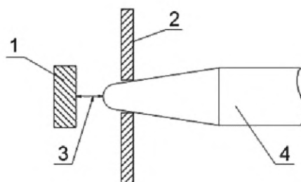
Рисунок 2С — Испытательный щуп
