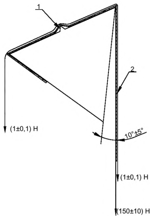
Рисунок АА.2 — Начальное положение оправки
