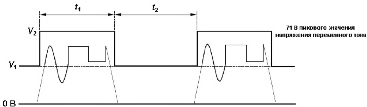
Рисунок 2Е.2 — Напряжения в БСНН цепях в условиях единичной неисправности при многократных импульсах выше V_1
