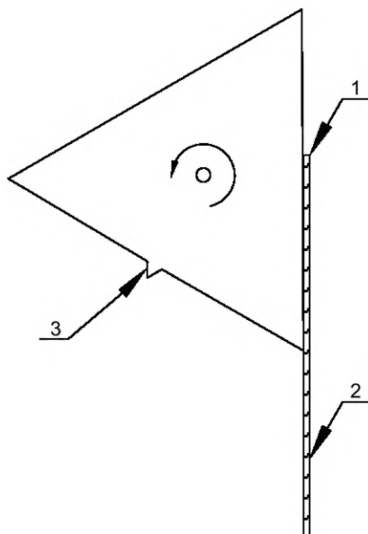
Рисунок АА.2 — Начальное положение оправки
