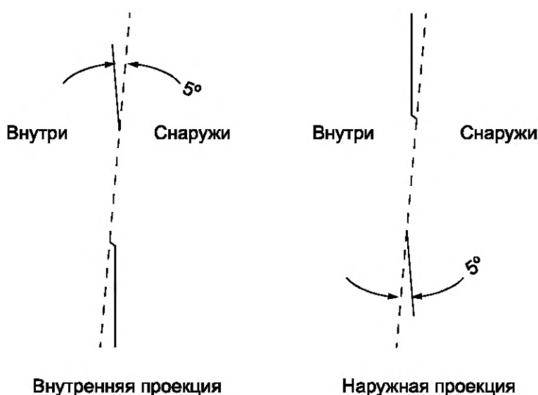
Рисунок 4С — Примеры конструкции жалюзи
