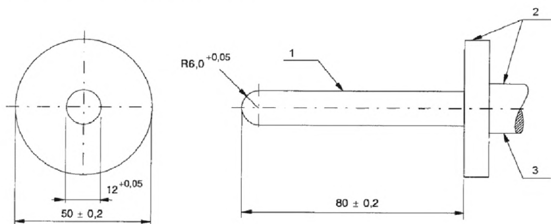
Рисунок 2С — Испытательный щуп
