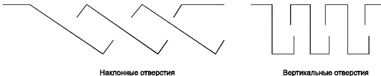
Рисунок 4В — Примеры поперечного сечения конструкции отверстий
