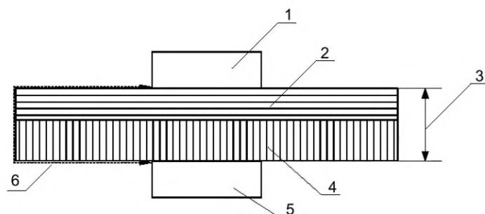
Рисунок F.14 — Сплошной изоляционный материал
