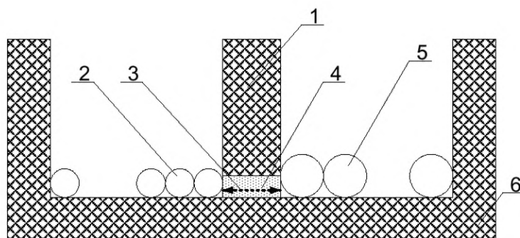
Рисунок F.17 — Компонент, заполненный изоляционным компаундом
