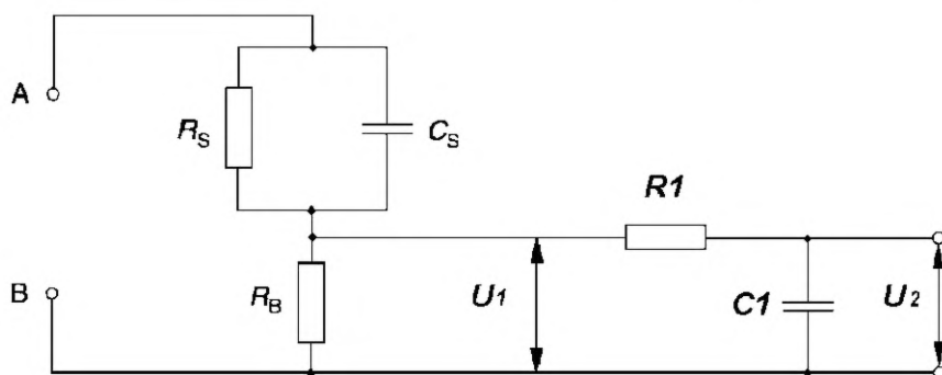
Рисунок D.1 — Измерительный прибор
