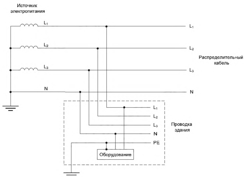
Рисунок V.5 — Пример ТТ-системы электропитания с тремя фазами и нейтралью
