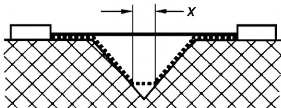
Рисунок F.3 — V-образная канавка
