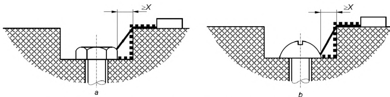
Рисунок F.9 — Широкое углубление
