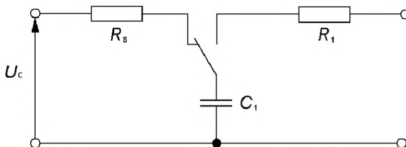
Рисунок N.2 — Схема испытательного генератора импульсов по IEC 60065
