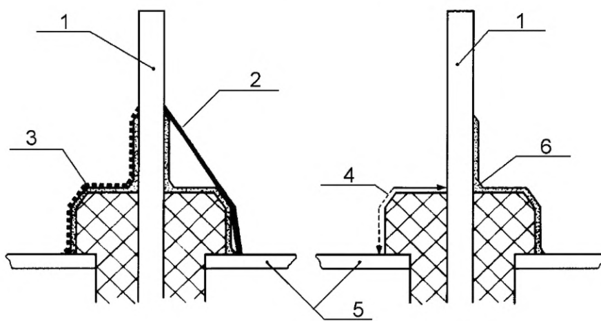
Рисунок F.9 — Широкое углубление
