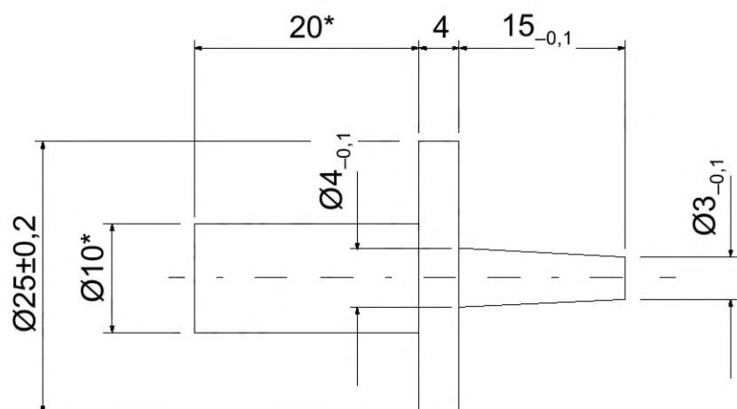
Рисунок 2В — Испытательный штырь
