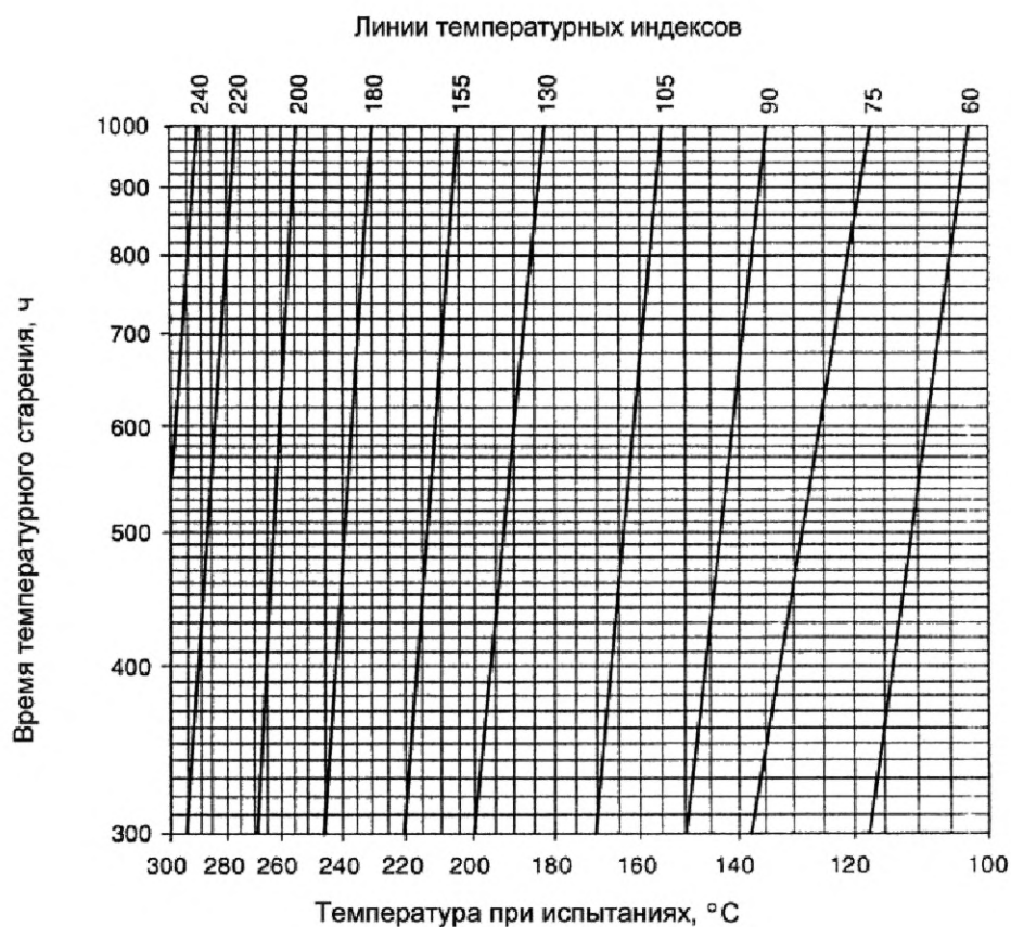
Рисунок 2J — Время теплового старения
