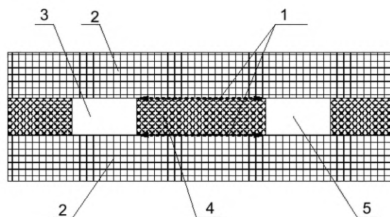
Рисунок F.15 — Тонколистовой изоляционный материал
