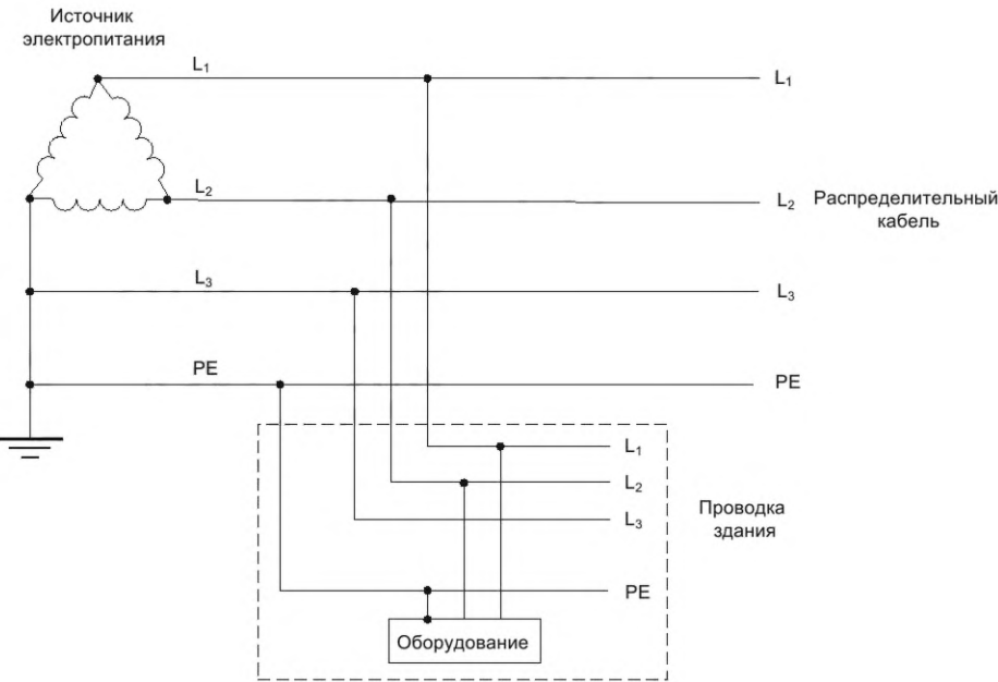
Заземленный проводник фазы
