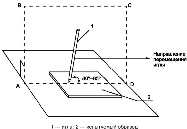
Рисунок 2К — Испытание покрывающего слоя на износостойкость
