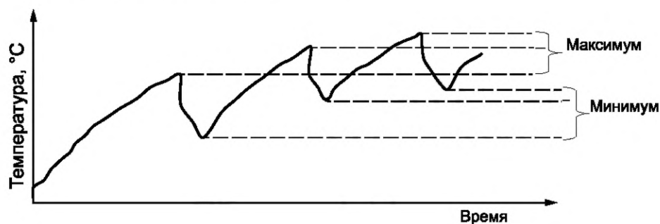
Рисунок В.1 — Определение среднеарифметического значения температуры
