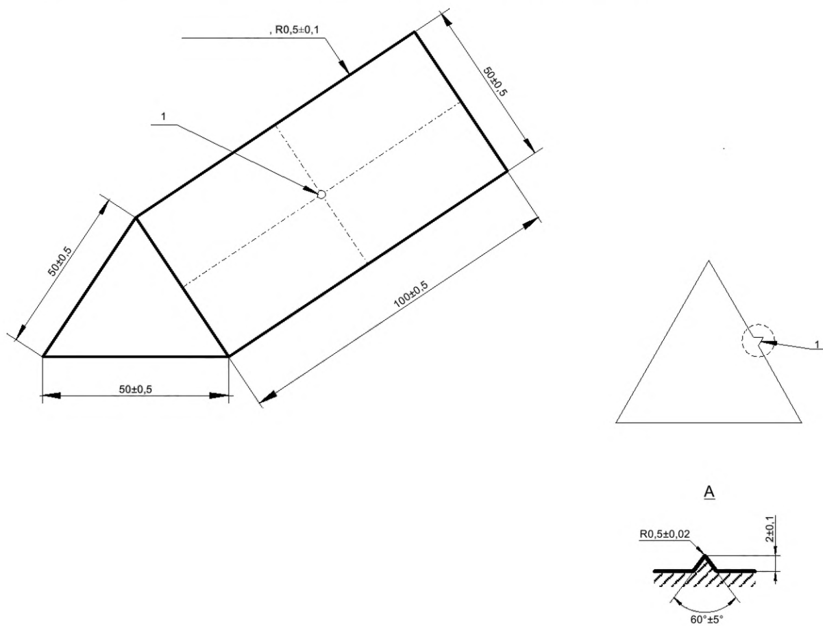
Рисунок АА.1 — Оправка
