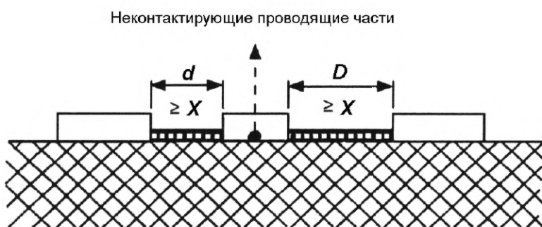
Рисунок F.13 — Интервал, несоединенная проводящая часть
