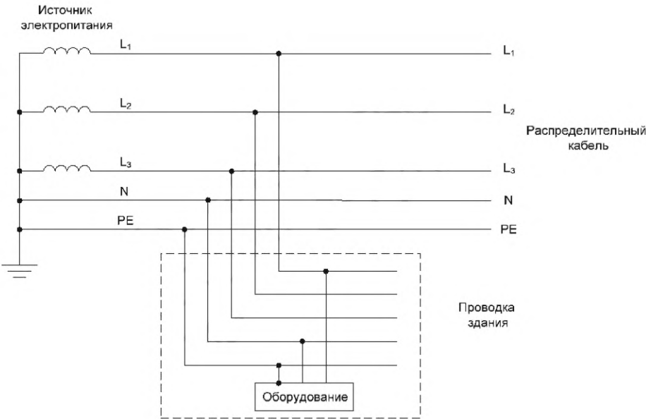
Разделенный нейтральный и защитный провода
