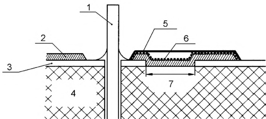
Рисунок F.10 — Покрытие вокруг выводов
