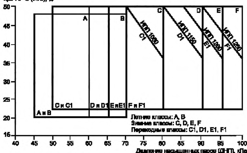
Объемная доля испарившегося бензина при 70 °C (И70), %
