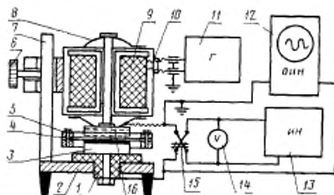
1—изолятор; 2—основание штатива; 3—нерподвижный электрод; 4—электрет; 5—корпус кассеты; 6—стопорный винт; 7—стойка штатива; 8—пружина; 9—катушка индуктивности; 10—экран катушки индуктивности; 11—генератор; 12—осциллографический индикатор нуля; 13—источник постоянного напряжения; 14—вольтметр; 15—переключатель полярности; 16—вибрирующий электрод
