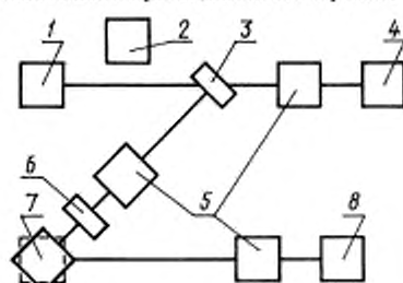
1 — вспомогательный лазер; 2 — средство юстировки; 3 — делительная пластина; 4 — измеритель энергии; 5 — оптическая система; 6 — ослабитель; 7 — фотометр сравнения; 8 — исследуемый лазер
