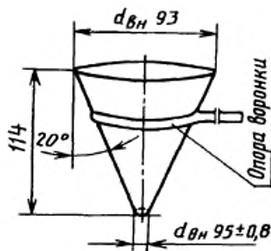
Испытательная воронка с опорой
