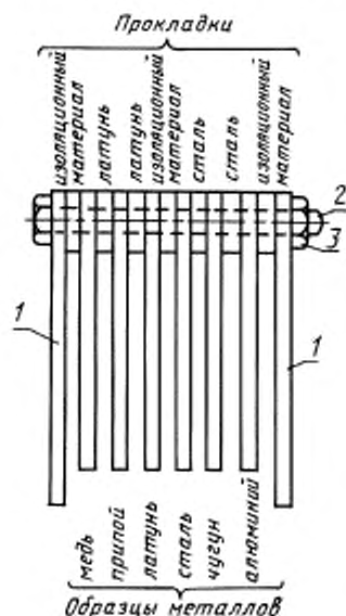
Держатель образцов металлов с набором пластин
