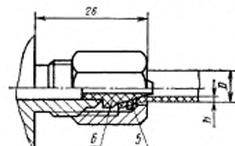
Исполнение 3 для пластмассовых труб
