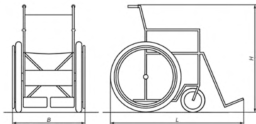
L — габаритная длина; B — габаритная ширина, H — габаритная высота
