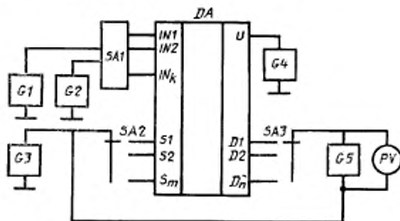
DA — измеряемая микросхема; S_1, S_2, \dots, S_m — аналоговые входы; D_1, D_2, \dots, D_n — аналоговые выходы; IN_1, IN_2, \dots, IN_k — управляющие входы; U — выход питания; G_1-G_4 — источники постоянного напряжения; G_5 — источник постоянного тока; SA_2, SA_3 — переключатели; SA_1 — коммутационное устройство, обеспечивающее подключение IN_1, IN_2, \dots, IN_k к G_1, G_2 ; PV — измеритель напряжения
