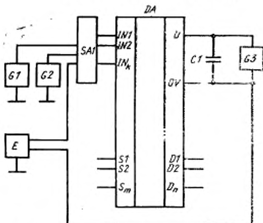
Схема измерения емкости управляющего входа
