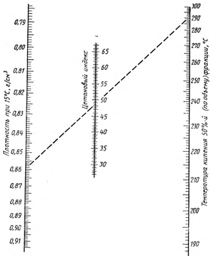
Номограмма для определения цетанового индекса (ЦИ)
