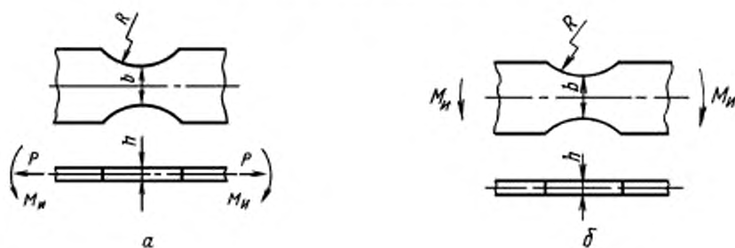
Рабочая часть образца типа III
