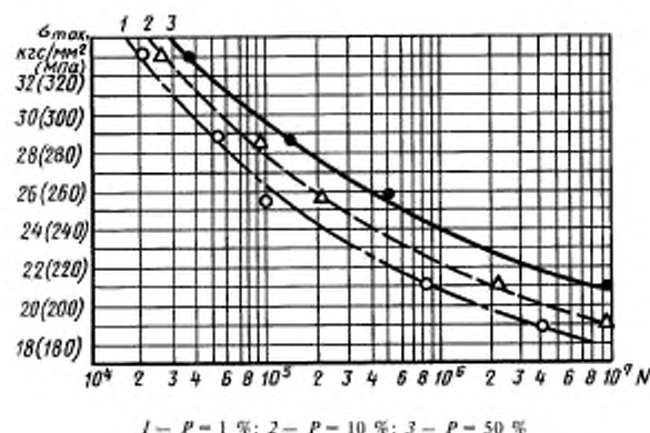
Кривые усталости образцов из сплава марки В95
