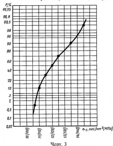
Кривая распределения предела ограниченной выносливости образцов из сплава марки АВ (база 5 \cdot 10^7 циклов)
