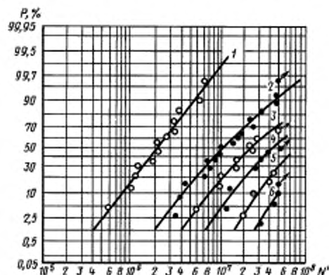
Кривые распределения долговечности образцов из сплава марки АВ
