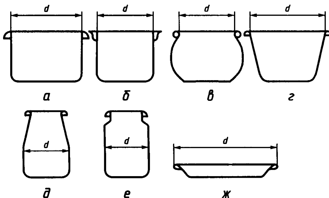
Схема измерения диаметров (габаритных размеров) посуды
