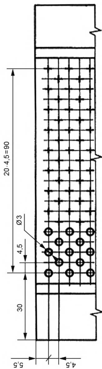
Рисунок 9 — Профили типа СА высотой 20 мм
