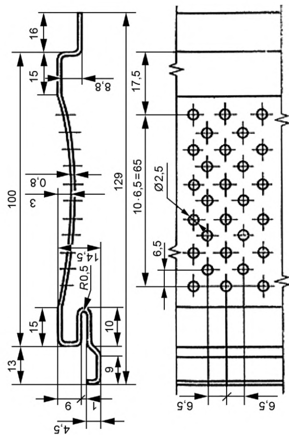
Рисунок 12 — Профили типа СА высотой 15 мм
