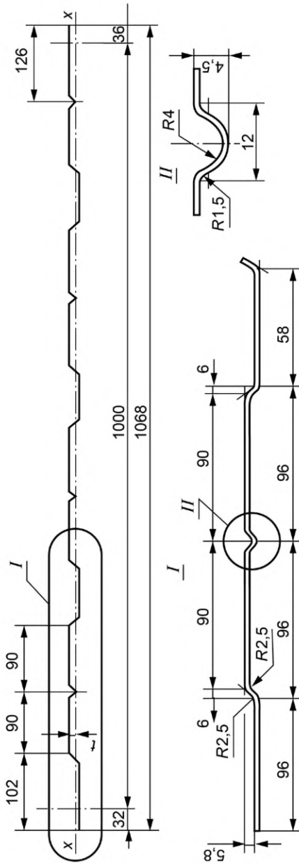
Рисунок 1 — Профили типа А высотой 6 мм
