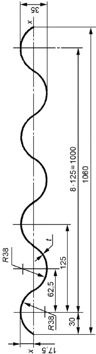
Рисунок 6 — Профили типа А высотой 35 мм
