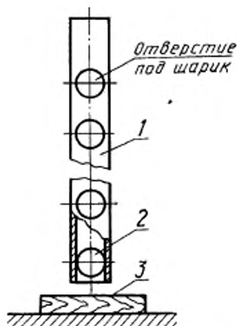
1 — направляющая труба; 2 — шарик; 3 — испытуемый образец
