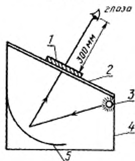
Схема приспособления для освещения пластинок
