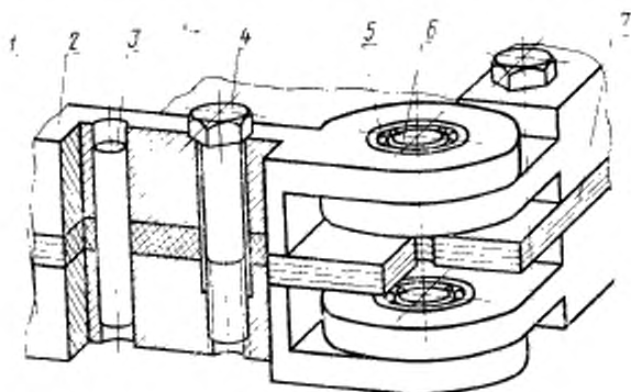
1, 2—четырёхзвёздник; 3—фиксатор; 4—болт; 5—подшипник радиальный; 6—ось вращения шарнира; 7—образец.
