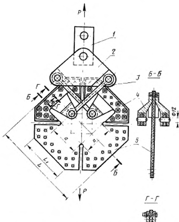
1—узел крепления в испытательной машине; 2—траверса; 3—тяга; 4—звено четырехзвенника (прижимные плашки); 5—образец
